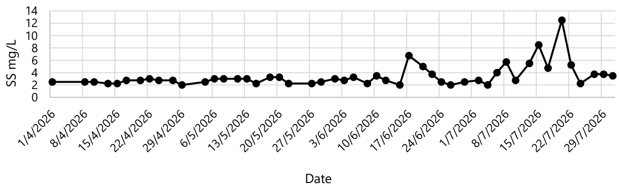
SS (Ebb)
